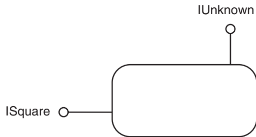
Abbildung 3.7: ISquare -Server in COM-Notation
